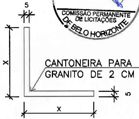
CANTONEIRA VISTA LATERAL E FRONTAL ESCALA: 1/20
