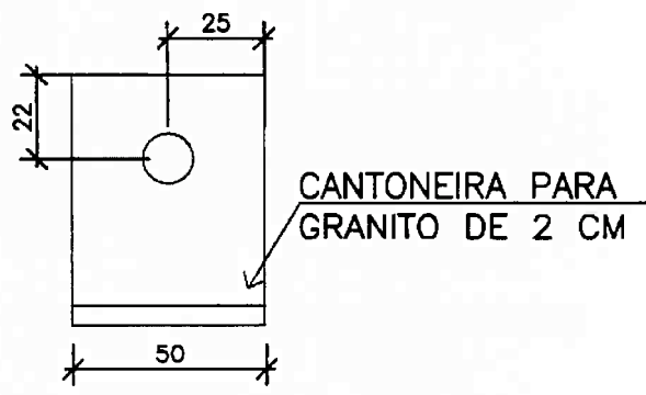
CANTONEIRA VISTA LATERAL E FRONTAL ESCALA: 1/20
